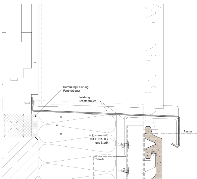
Brüstung mit Anschluss Fensterbank
