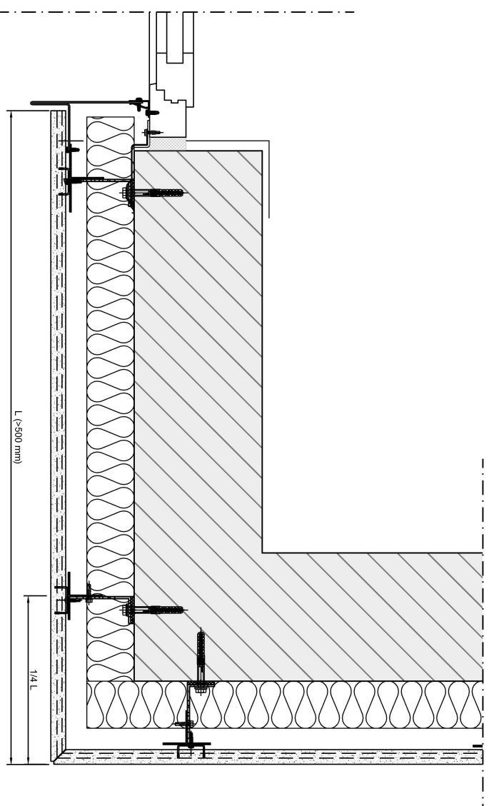
D1 - Fugen mit Fugenprofil
