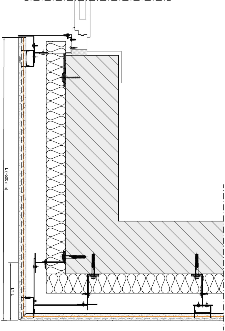
D1 - Fugen mit Fugenprofil
