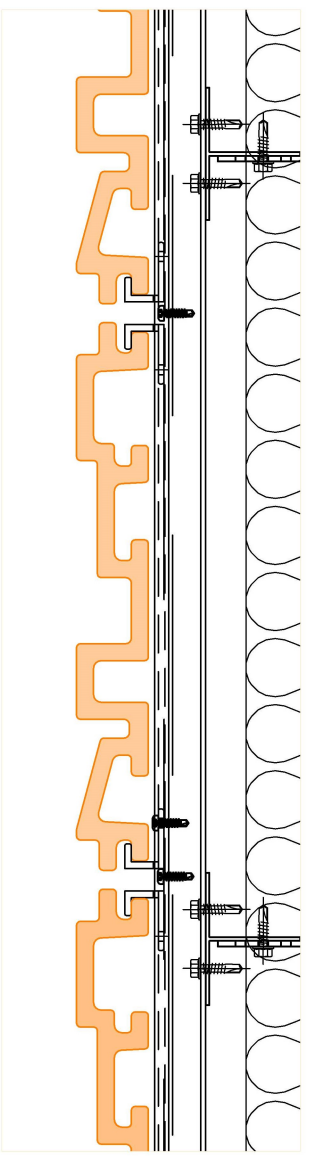
D1 - Befestigung der Fassadenelemente
