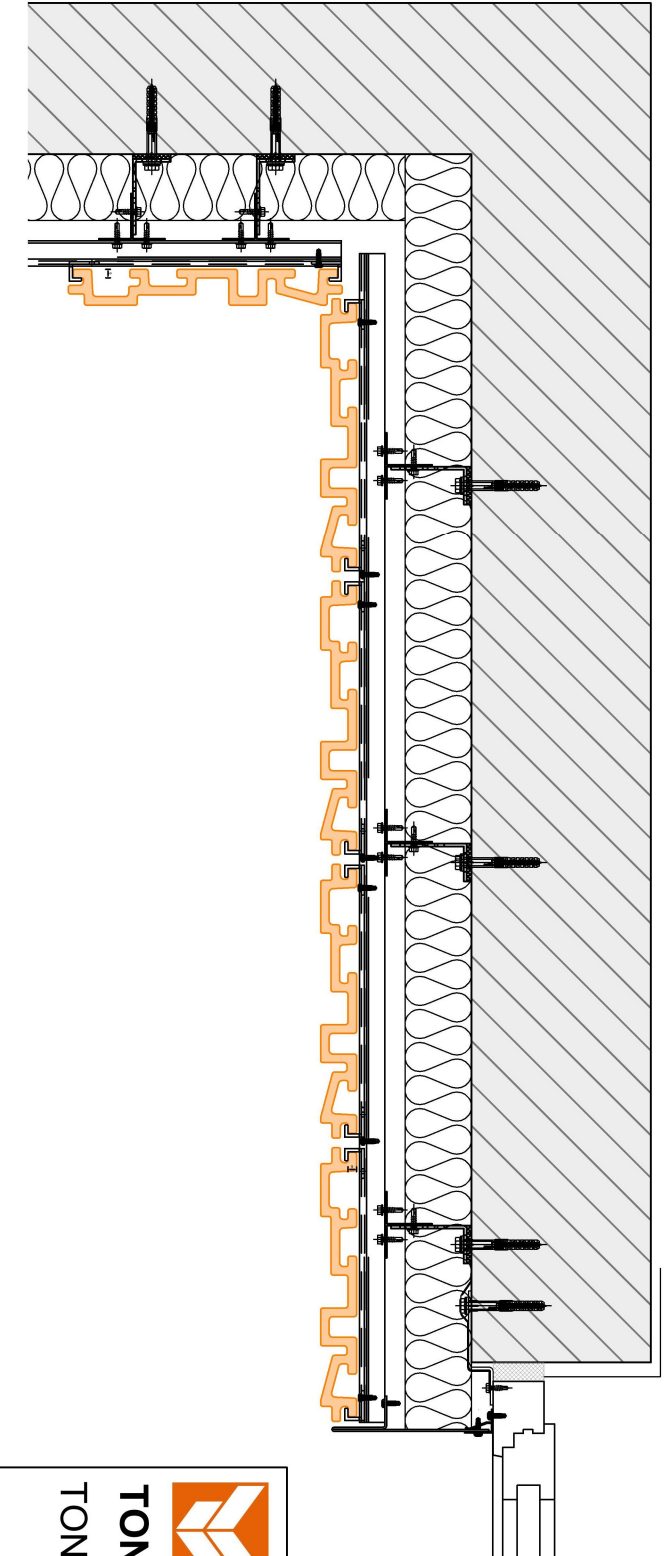
TON-V-UK - Einzelteile
