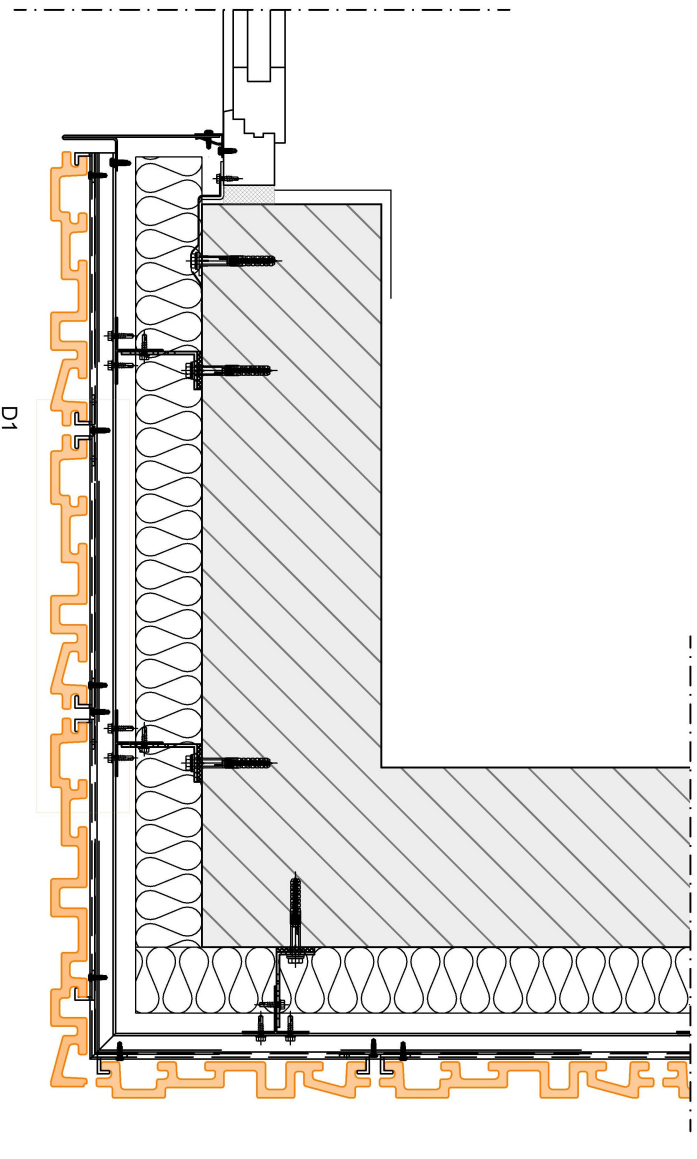
D1 - Befestigung der Fassadenelemente
