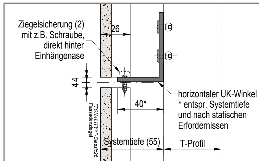
Vertikaldetail zu Ziegelsicherung (2)
